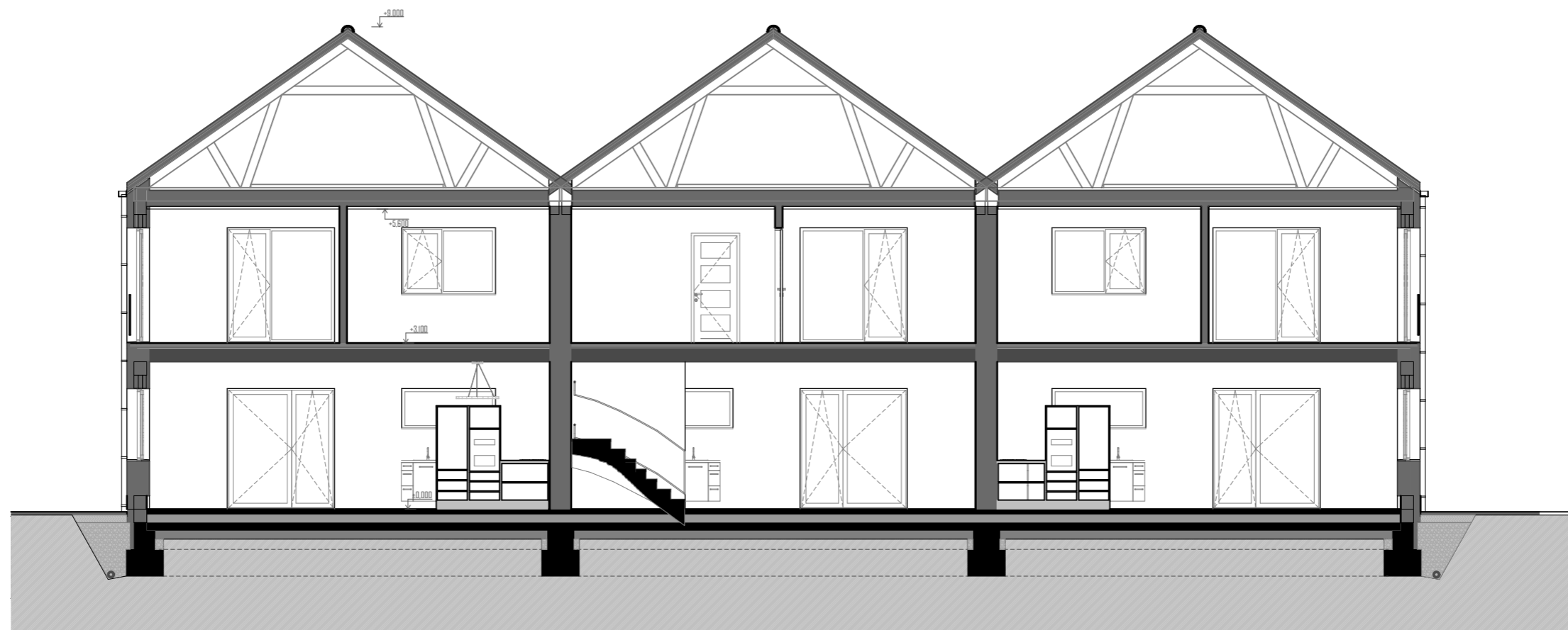
ŘEZ PŘÍČNÝ
